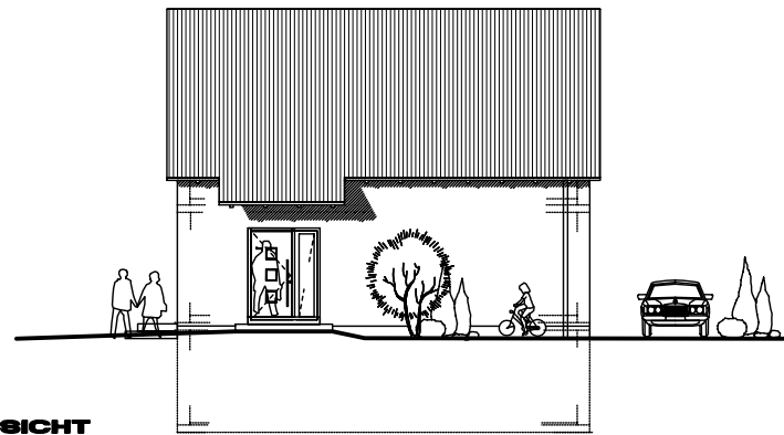
WEST ANSICHT
