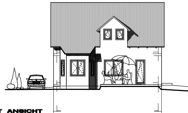
OST ANSICHT
