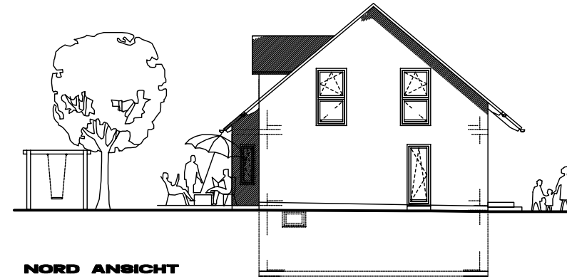
NORD ANSICHT
