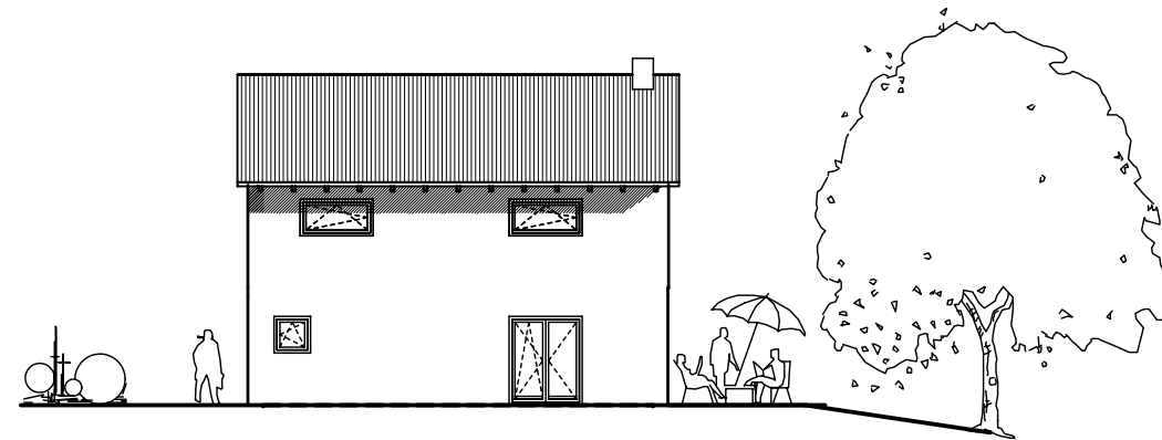
NORD ANSICHT
